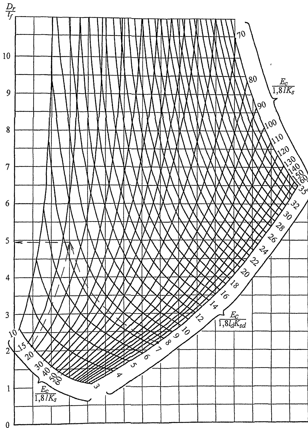
Рисунок М.2 – Номограмма для определения отношения \frac{D_r}{t_f}
