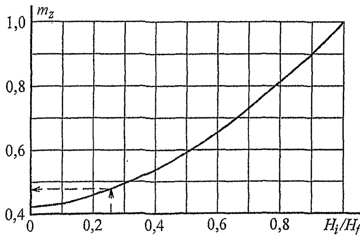
Рисунок Е.2 – График для определения коэффициента m_z
