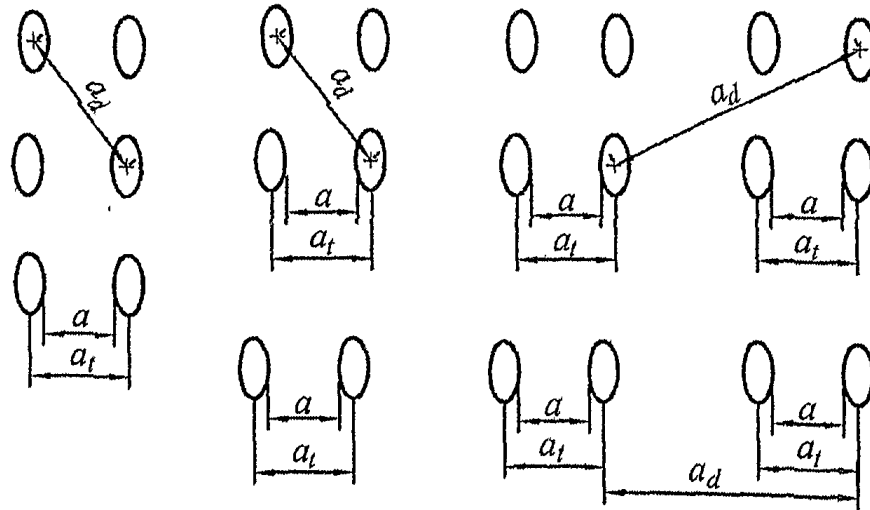
Рисунок К.7 – Расчетные расстояния a , a_l , a_d между колесами опор воздушных судов
