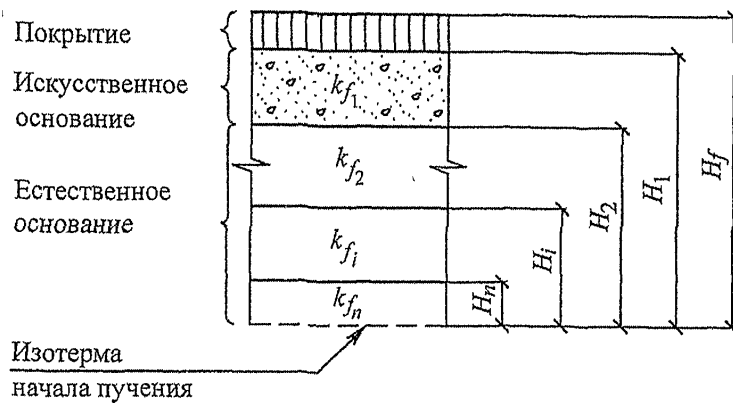
Рисунок Е.1 – Расчетная схема слоистого основания
